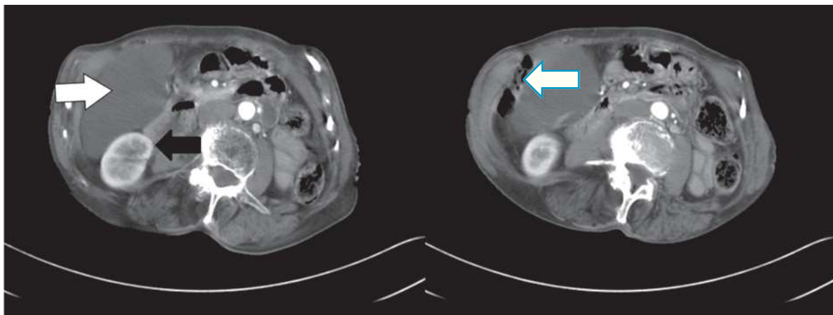
■ Figura 1. TC de abdomen que muestra una lesión retroperitoneal quística por debajo del hígado (flecha blanca), delante del riñón derecho (flecha negra) y por detrás del colon derecho, (flecha en marco azul) de aproximadamente 14 cm por 12 cm y 14 UH.
