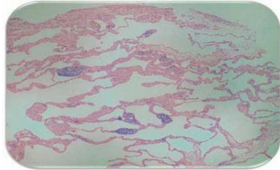
■ Figura 3. Vista microscópica del linfangioma quístico retroperitoneal constituida por múltiples canales vasculares linfáticos de diversas formas y tamaño, revestidos por endotelio y grupos de linfocitos.
