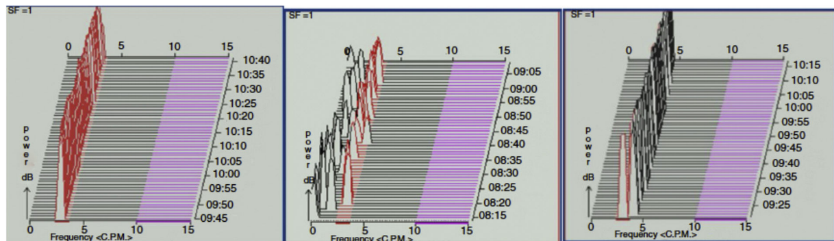
Figura 1 Registros de electrogiografía de superficie. Frecuencia de rangos de ondas lentas gástricas: A) normal entre 2.4 y 3.7 cpm. B) Bradigastria entre 0.5 y 2.3 cpm. C) Taquigastria entre 3.8 y 10 cpm. Cada línea representa un minuto de análisis.
